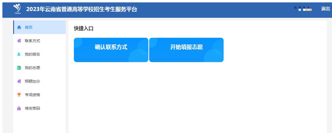
图 3.1 考生首页
